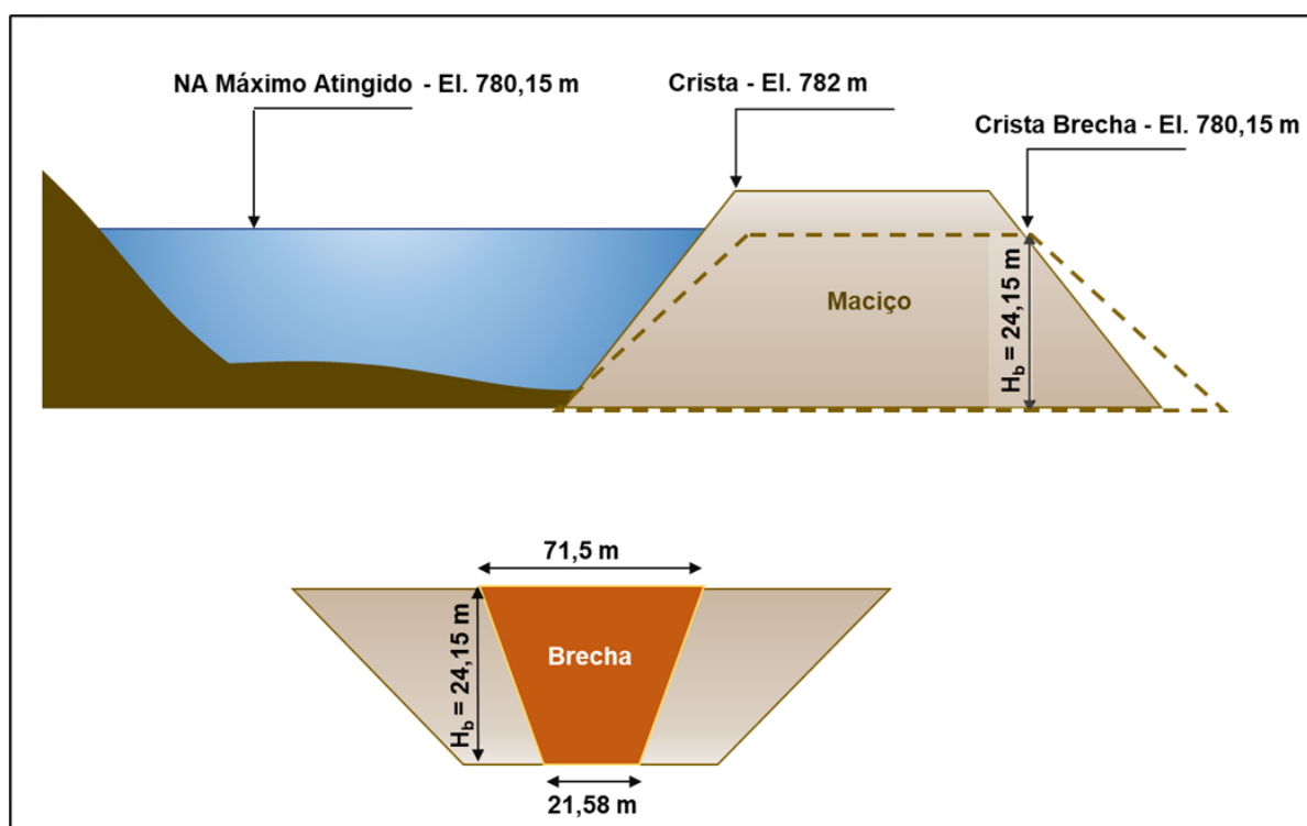
Figura 10-1 – Parâmetros da brecha de ruptura.
