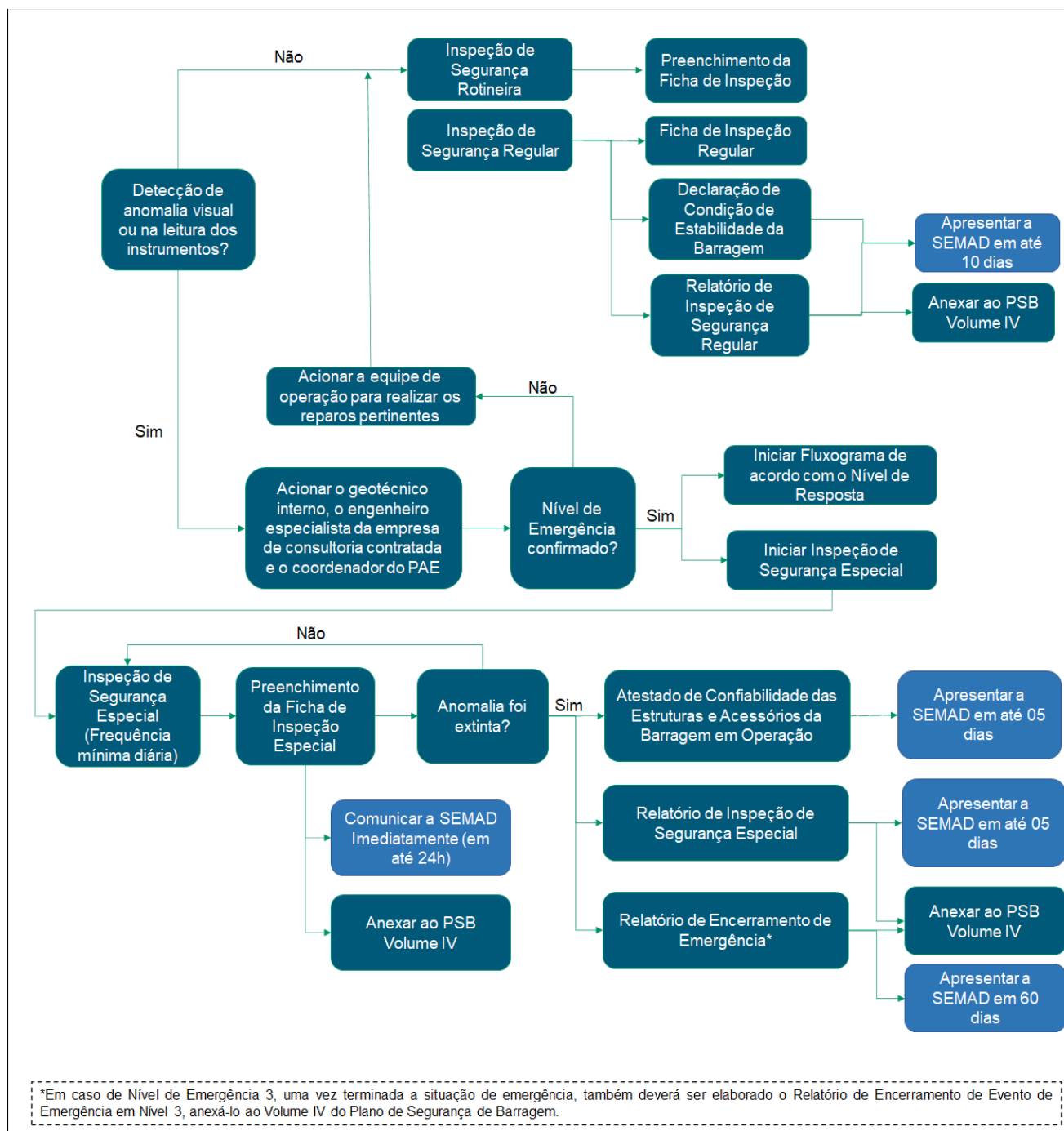
Figura 6-2 – Processo de detecção de uma situação de emergência e relatórios associados.
