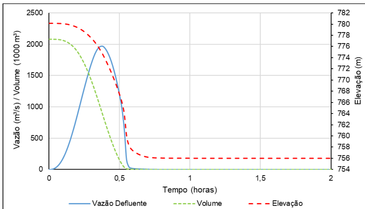
Figura 10-2 - Hidrograma de ruptura - Barragem do Mosquito.
