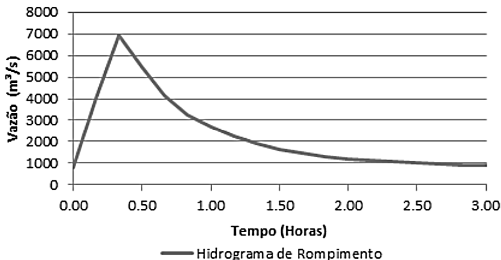
Figura 12. Hidrograma de rompimento da barragem – UHE Porto Raso.
