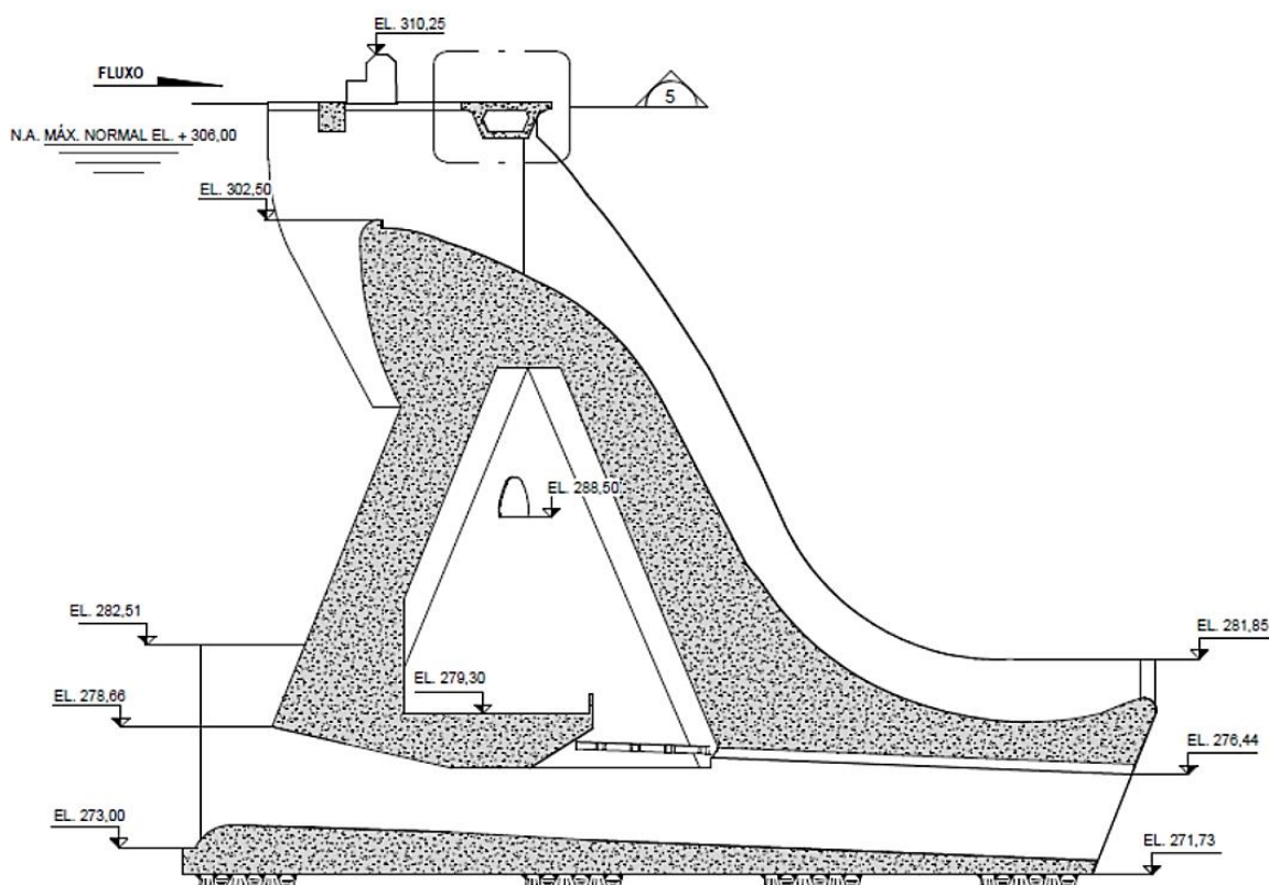
Figura 7. Vertedouro de Superfície e Descarregador de Fundo da UHE Porto Raso.
