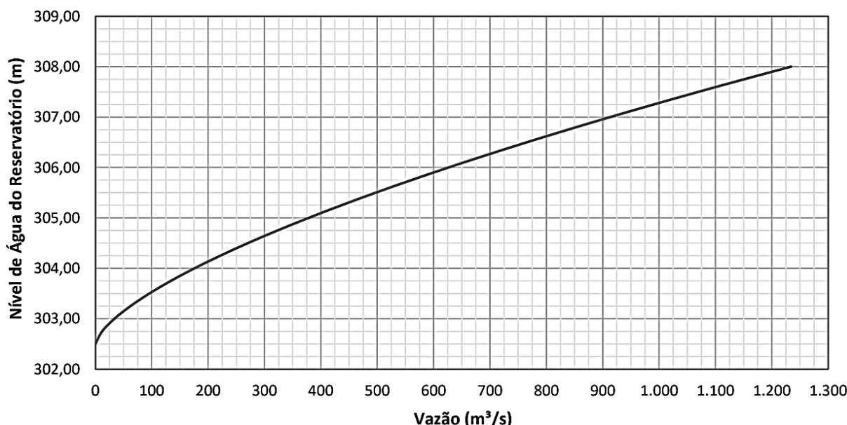
Figura 8. Curva de Descarga do Vertedouro de Superfície – UHE Porto Raso.
