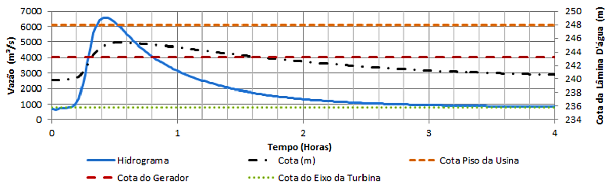
Figura 13. Hidrograma e cotagrama do rio Juquiá junto à casa de força da UHE Porto Raso após a ruptura da barragem da UHE.
