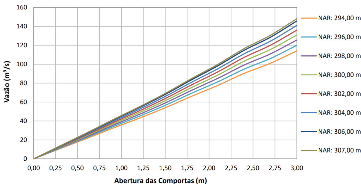
Figura 9. Curvas de Descarga do Descarregador de Fundo para diferentes Níveis de Água do Reservatório – UHE Porto Raso.
