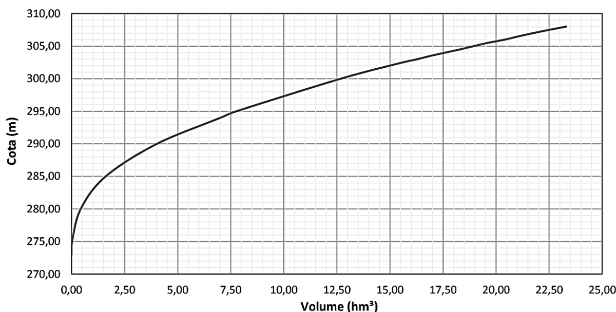
Figura 5. Curva cota x volume do reservatório – UHE Porto Raso.
