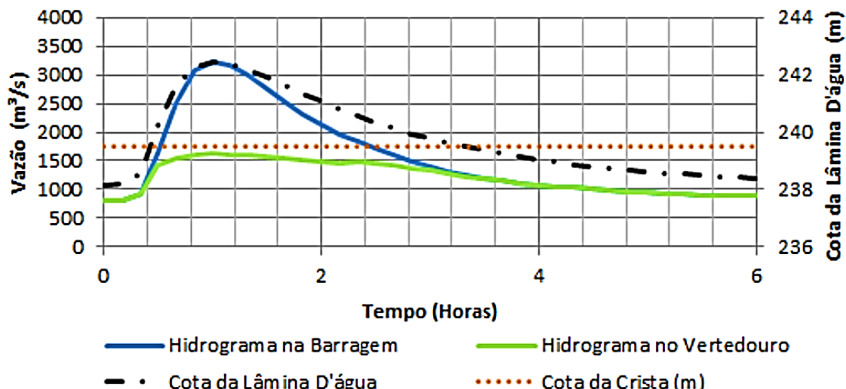
Figura 14. Hidrograma e cotograma do rio Juquiá junto à barragem da UHE Alecrim após a ruptura da barragem da UHE Porto Raso.
