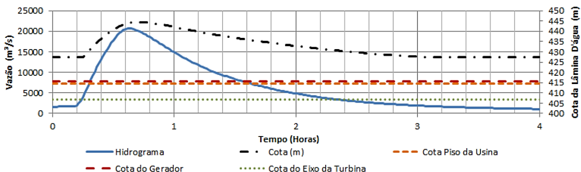
Figura 16. Hidrograma e cotograma do rio Juquiá junto à casa de força da UHE Fumaça após a ruptura da barragem da UHE.
