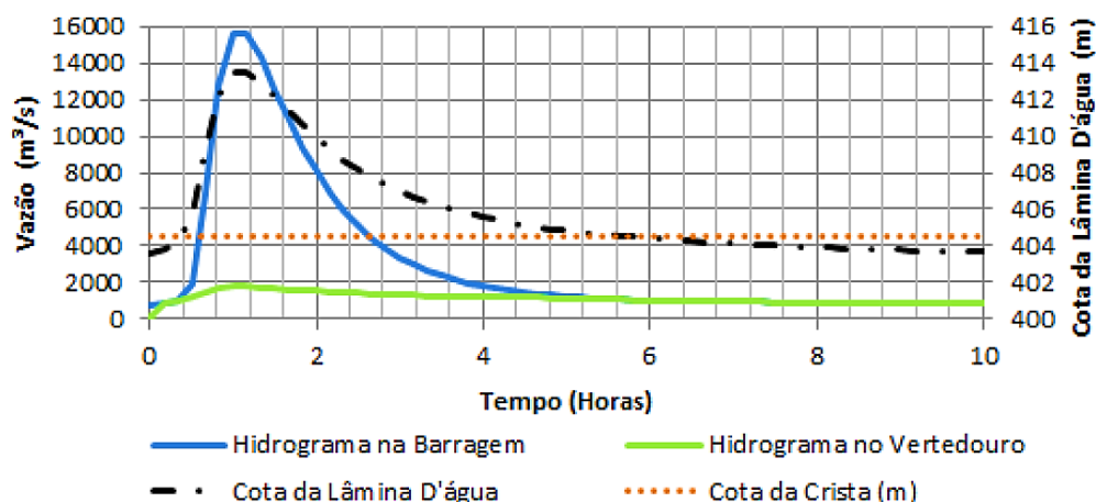
Figura 17. Hidrograma e cotograma do rio Juquiá junto à barragem da UHE Barra após a ruptura da barragem da UHE Fumaça.
