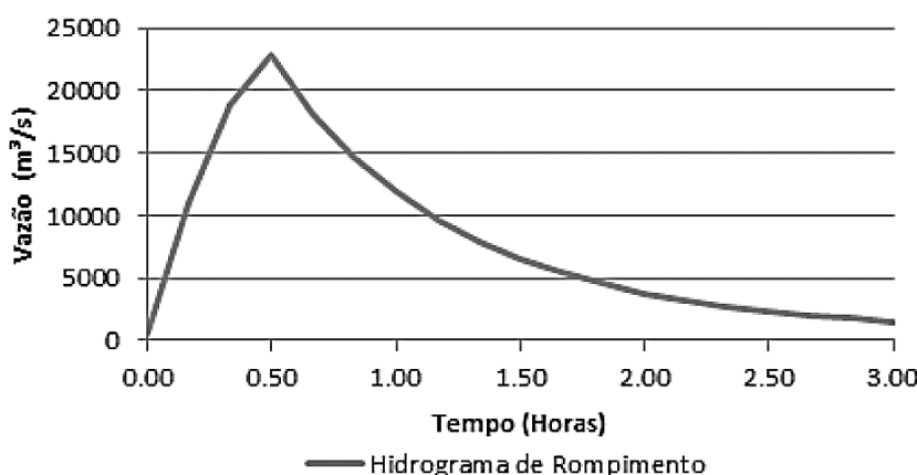
Figura 15. Hidrograma de rompimento da barragem – UHE Fumaça.
