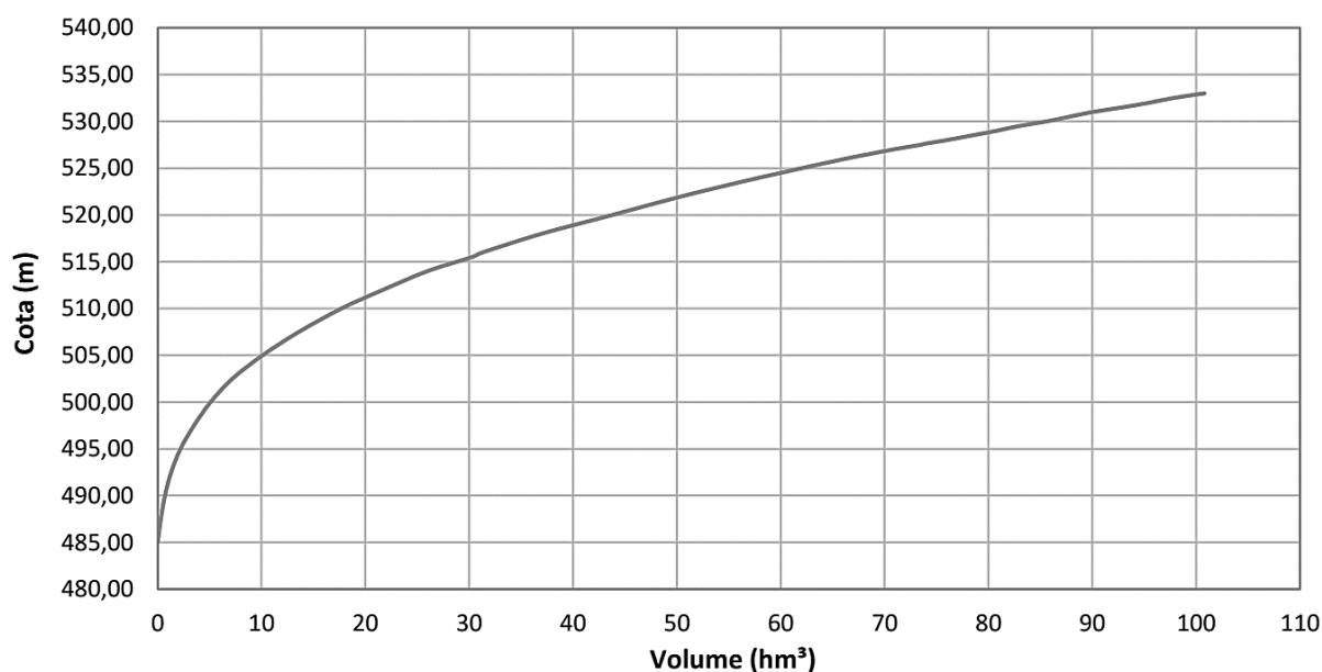
Figura 5. Curva cota x volume do reservatório – UHE Fumaça Fonte: CV1901-FUM-RP04-RT-0001-00 (VLB ENGENHARIA, 2021)
