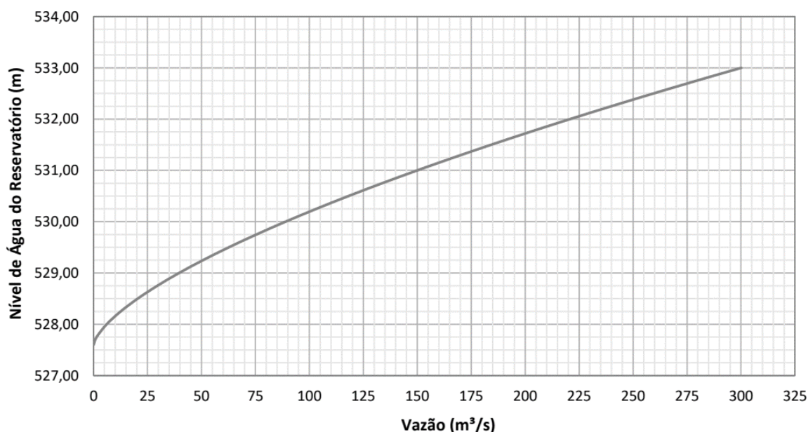
Figura 10. Curva de Descarga do Vertedouro de Superfície com Comporta Plana – UHE Fumaça.
