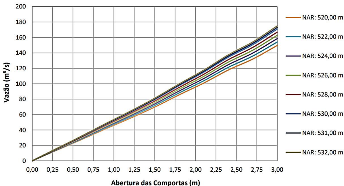
Figura 12. Curvas de Descarga do Descarregador de Fundo para diferentes Níveis de Água do Reservatório – UHE Fumaça.
