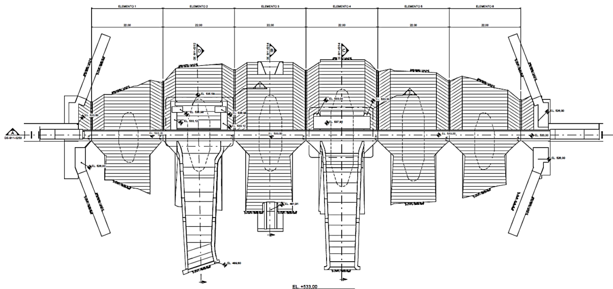
Figura 8. Planta da Barragem da UHE Fumaça.
