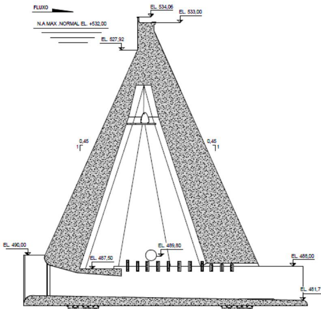
Figura 11. Corte do Descarregador de Fundo e Elemento 3 da Barragem da UHE Fumaça.
