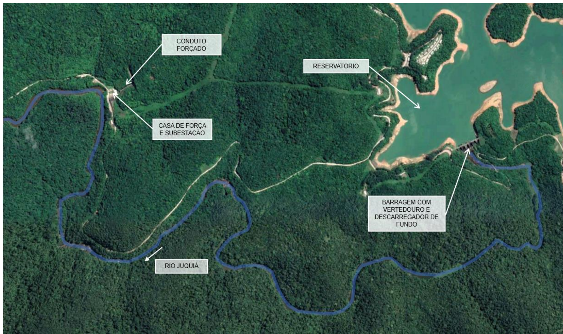
Figura 1. UHE Fumaça – Arranjo Geral - Planta.
