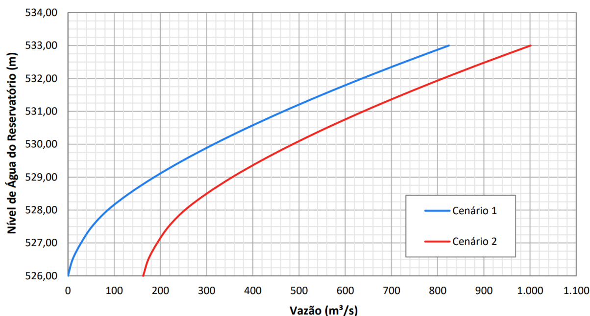
Figura 13. Curva de Descarga para o Cenário de Operação Conjunta das Estruturas Extravasoras – UHE Fumaça.
