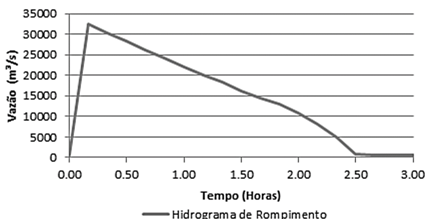
Figura 14. Hidrograma de rompimento da barragem – UHE França.
