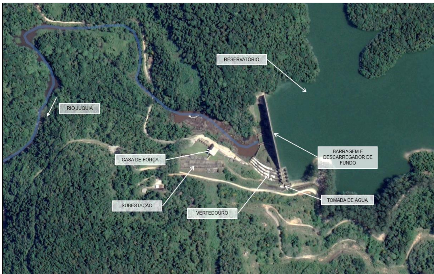
Figura 1. UHE França – Arranjo Geral - Planta.
