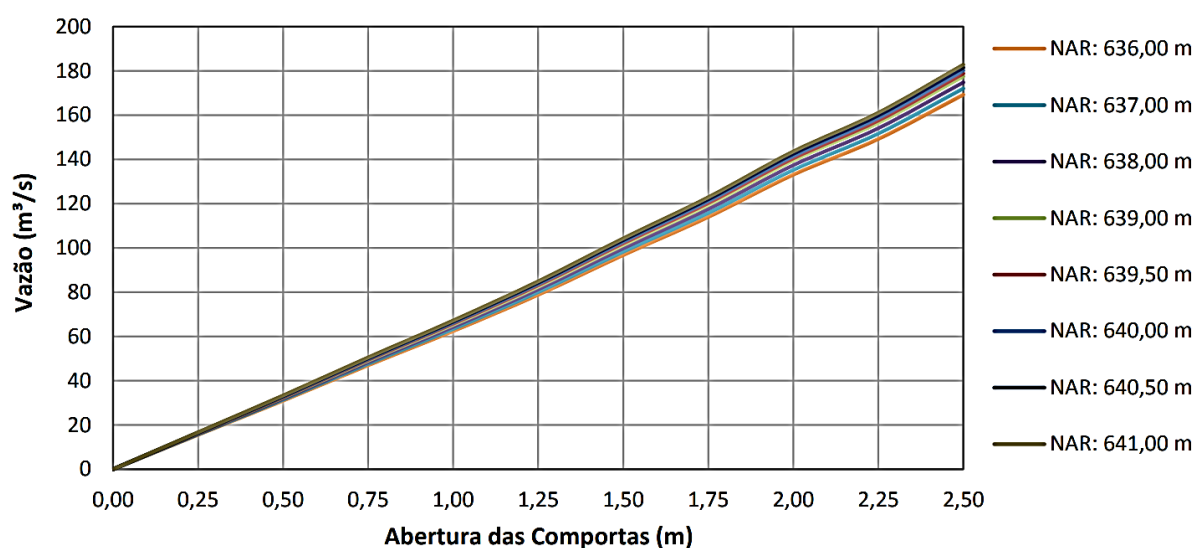
Figura 11. Curvas de Descarga do Descarregador de Fundo para diferentes Níveis de Água do Reservatório – UHE França.
