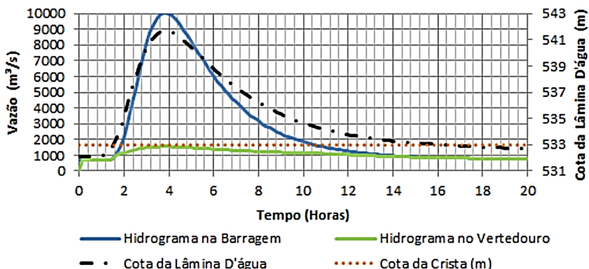
Figura 15. Hidrograma e cotagrama imediatamente a montante da barragem da UHE Fumaça após a ruptura da barragem da UHE França.
