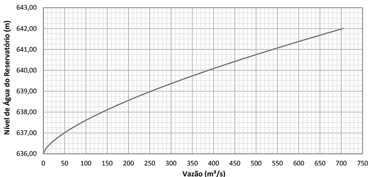
Figura 10. Curva de Descarga do Vertedouro de Superfície – UHE França.
