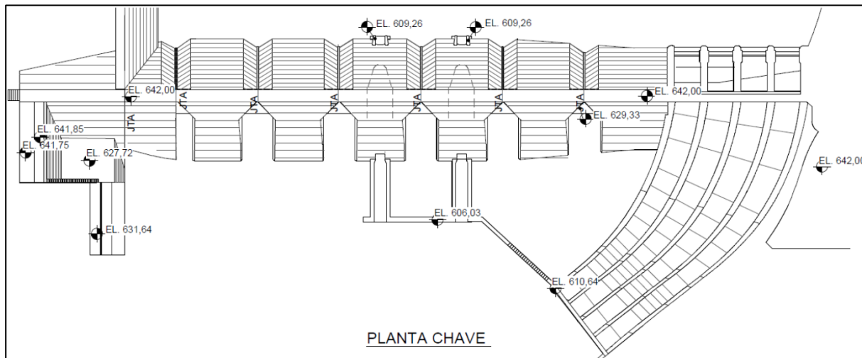
Figura 7. Planta da Barragem da UHE França indicando o Vertedouro de Superfície e os dois Descarregadores de Fundo.
