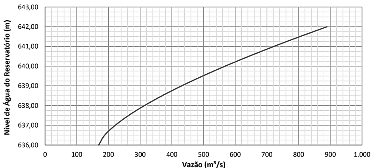
Figura 12. Curva de Descarga para o Cenário de Operação Conjunta das Estruturas Extravasoras – UHE França.
