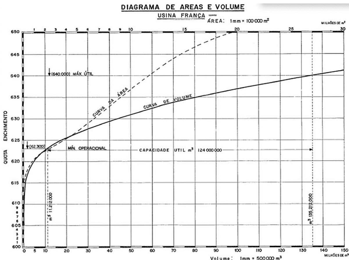
Figura 5. Curva cota x volume do reservatório – UHE França.
