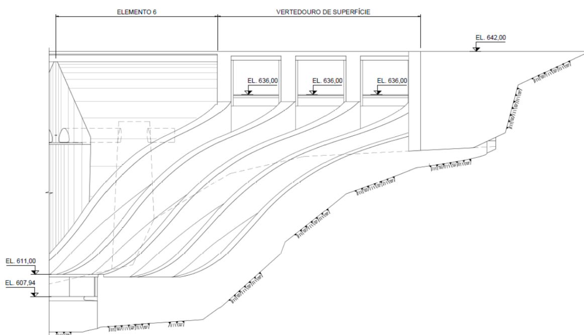
Figura 9. Vista de jusante do Vertedouro de Superfície da UHE França (projeto).
