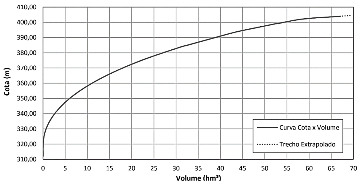
Figura 5. Curva cota x volume do reservatório – UHE Barra.
