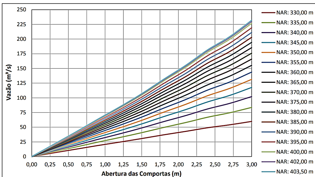
Figura 11. Curvas de Descarga do Descarregador de Fundo para diferentes Níveis de Água do Reservatório – UHE Barra.
