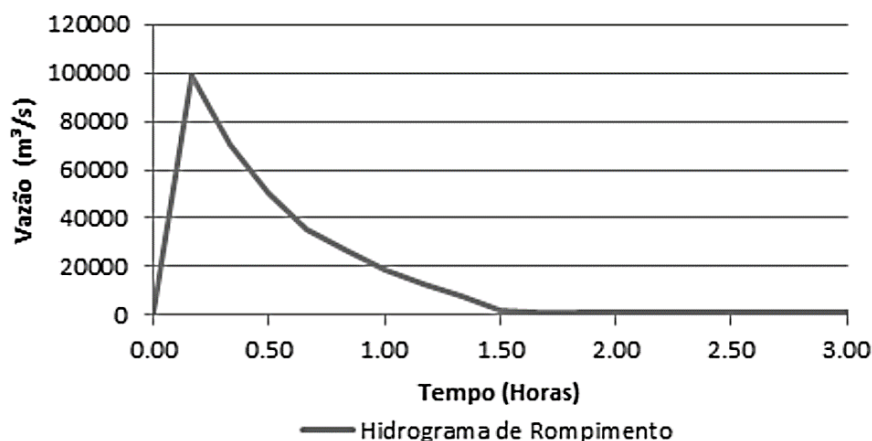
Figura 14. Hidrograma de rompimento da barragem – UHE Barra.
