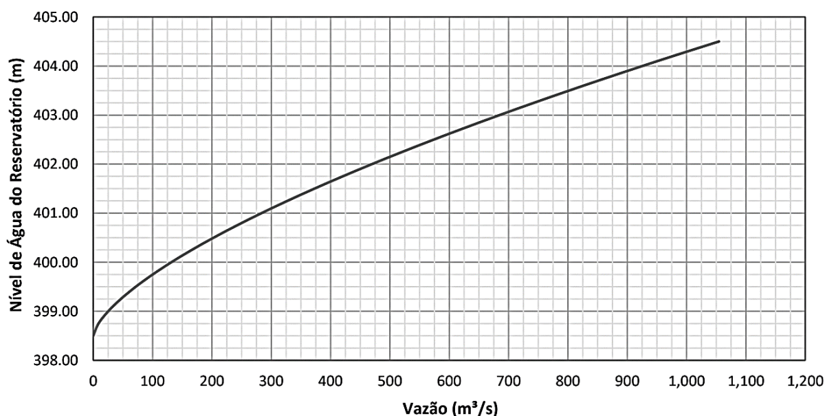
Figura 9. Curva de Descarga do Vertedouro de Superfície – UHE Barra.
