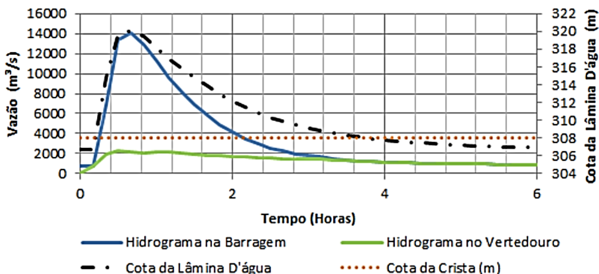
Figura 15. Hidrograma e cotagrama do rio Juquiá na barragem da UHE Porto Raso após a ruptura da barragem da UHE Barra.
