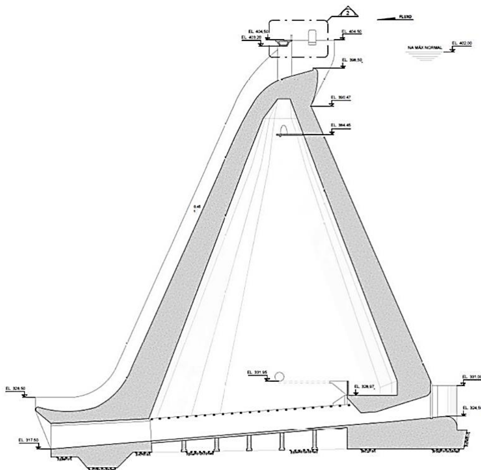
Figura 7. Vertedouro de Superfície e Descarregador de Fundo da UHE Barra.
