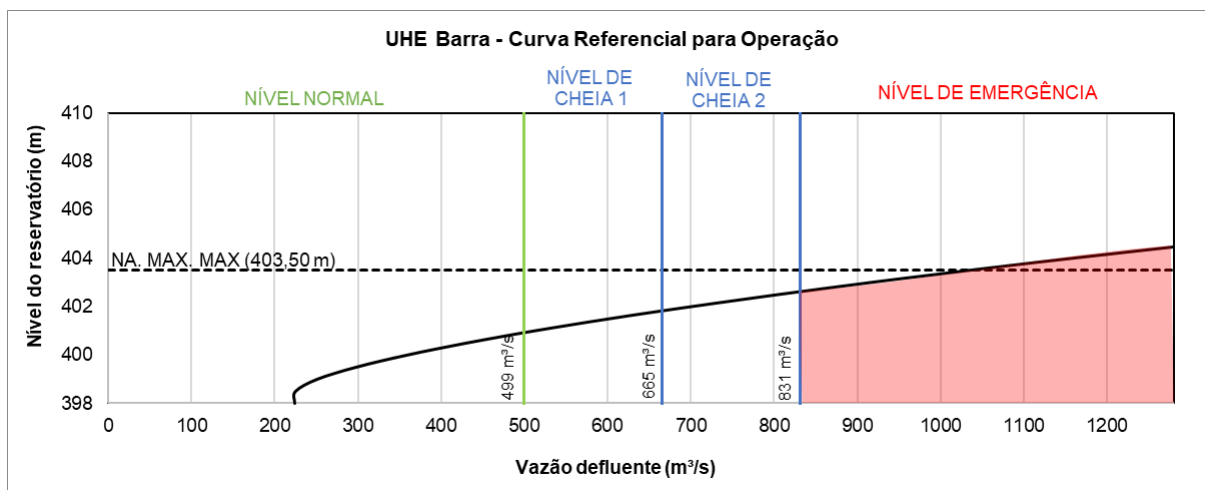
Figura 13. Nível de Resposta hidrológica.
