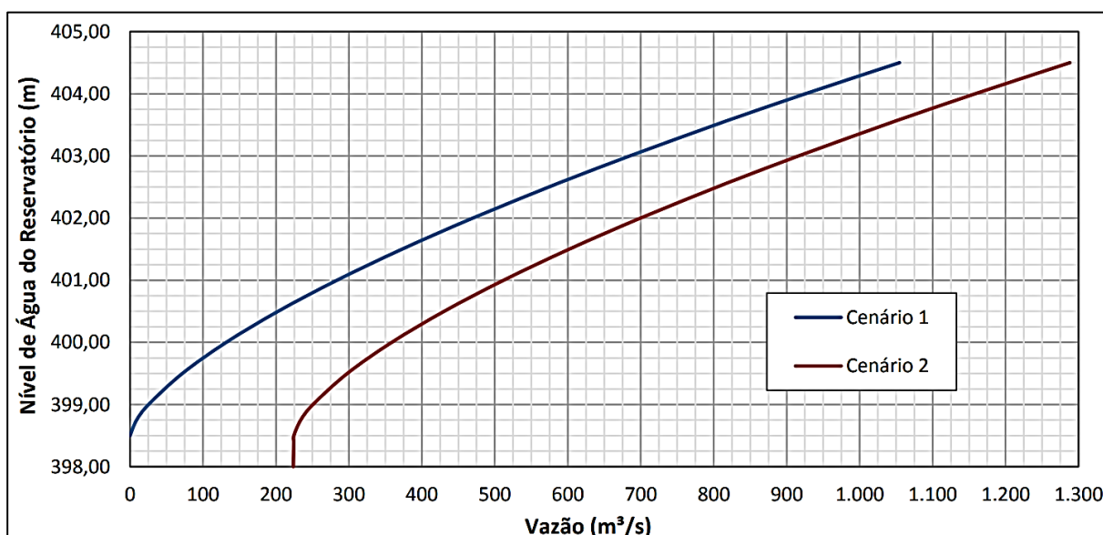
Figura 12. Curva de Descarga para o Cenário de Operação Conjunta das Estruturas Extravasoras – UHE Barra.
